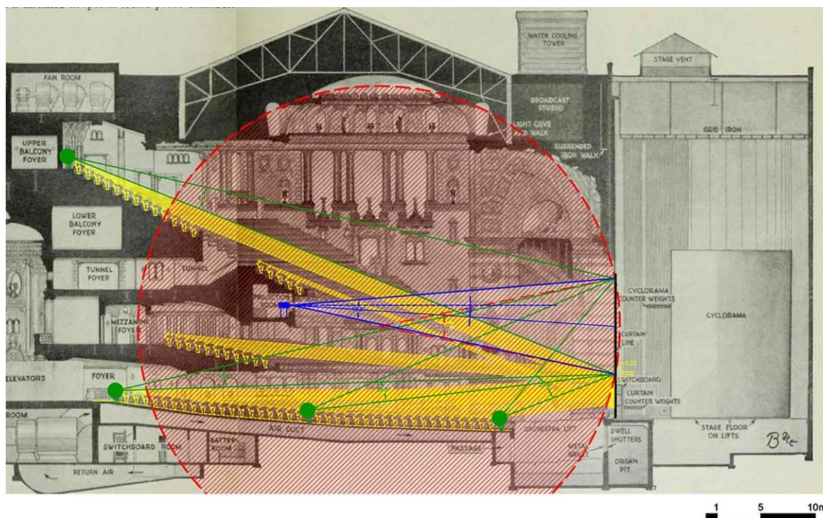
Εικ 4. Roxy Theater [Izenour, 1996], έλεγχο οπτικής άνεσης σε αξονική τομή
